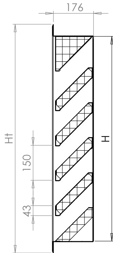
SECTION A-A
